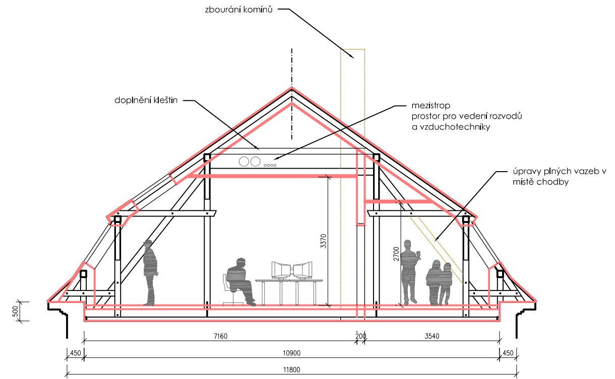
ŘEZ B-B
