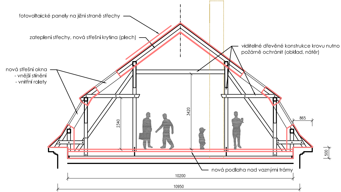
ŘEZ A-A
